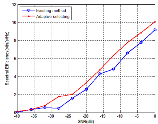
그림 4. 제안하는 알고리즘의 SNR 값에 따른 스펙트럼 효율 성능 비교 그래프
