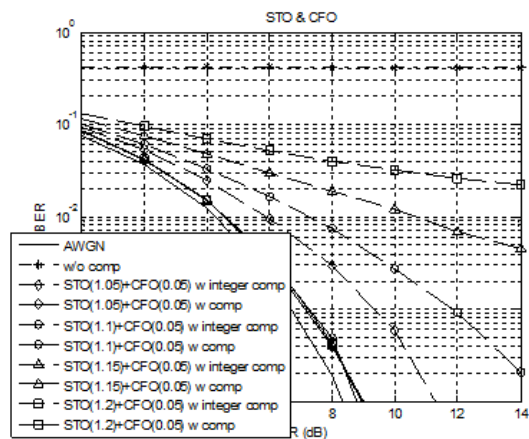
그림 8. STO와 CFO의 보상 성능. Fig. 8. BER performance at joint environment with STO and CFO.
