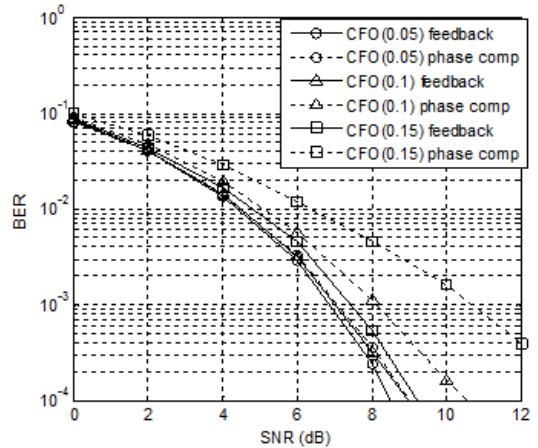
그림 9. Feedback 방식을 이용한 시간영역 보상과 Feedback을 하지 않은 주파수영역 보상의 차이 Fig. 9. BER performance of different compensation methods between time and frequency domain.
