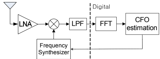
그림 3. Fractional PLL을 이용한 CFO 정정. Fig. 3. Correction of CFO using fractional PLL
