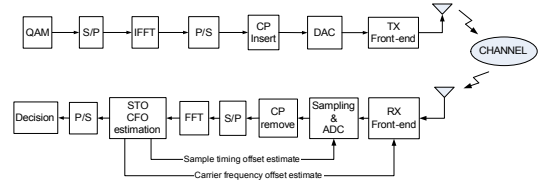
그림 2. OFDM 시스템 모델. Fig. 2. OFDM system model.
