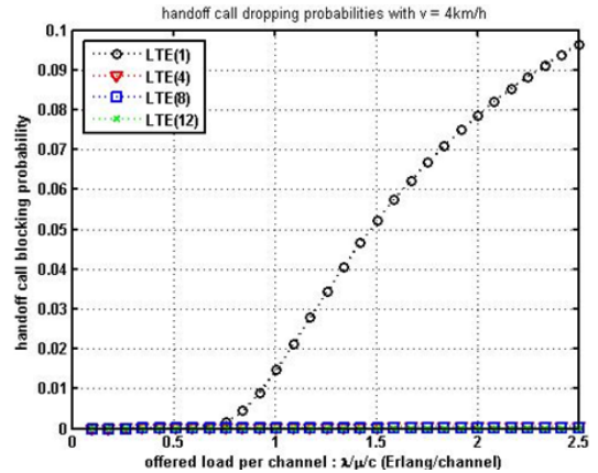
그림 12. RB 당 offered load에 따른 핸드오프호 절단률 ( v=4\text{km/h} , Guard RB 변화, P=P^*=1 )
