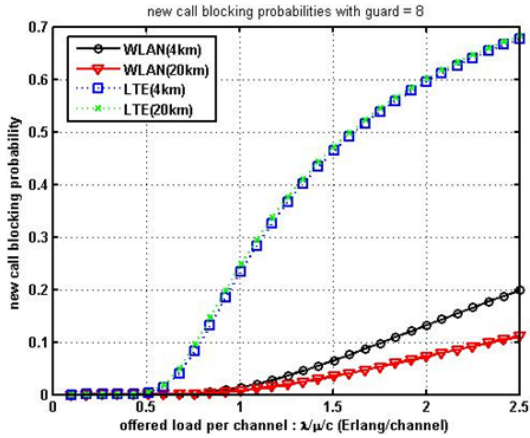
그림 6. RB 당 offered load에 따른 네트워크 별 신규호 차단률(JCAC 적용 모델)
