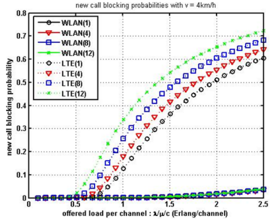
그림 8. RB 당 offered load에 따른 네트워크 별 신규호 차단률( v=4\text{km/h} , Guard RB 변화, P=P^*=1/2 )
