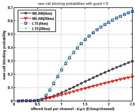
그림 7. RB 당 offered load에 따른 네트워크 별 신규호 차단률(Non-JCAC 적용 모델)
